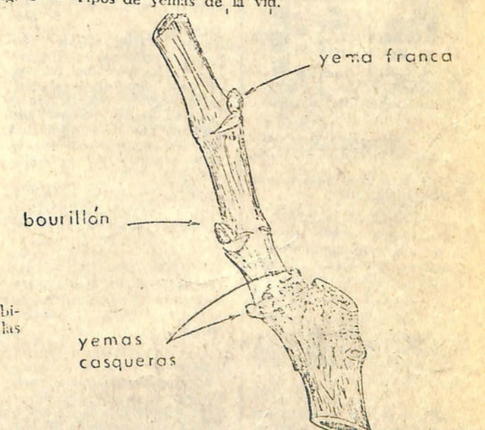
Fig. 1 — Tipos de yemas de la vid.
