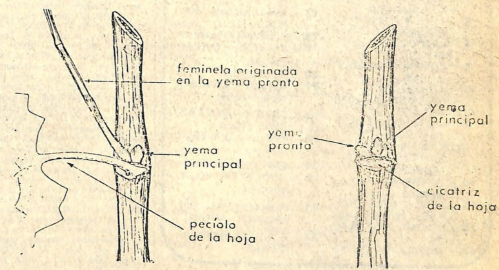
Fig. 1 — Tipos de yemas de la vid.
