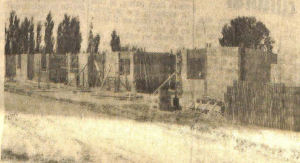
En la fotografía se observan siete viviendas con mampostería encadenada superior, sobre un...
