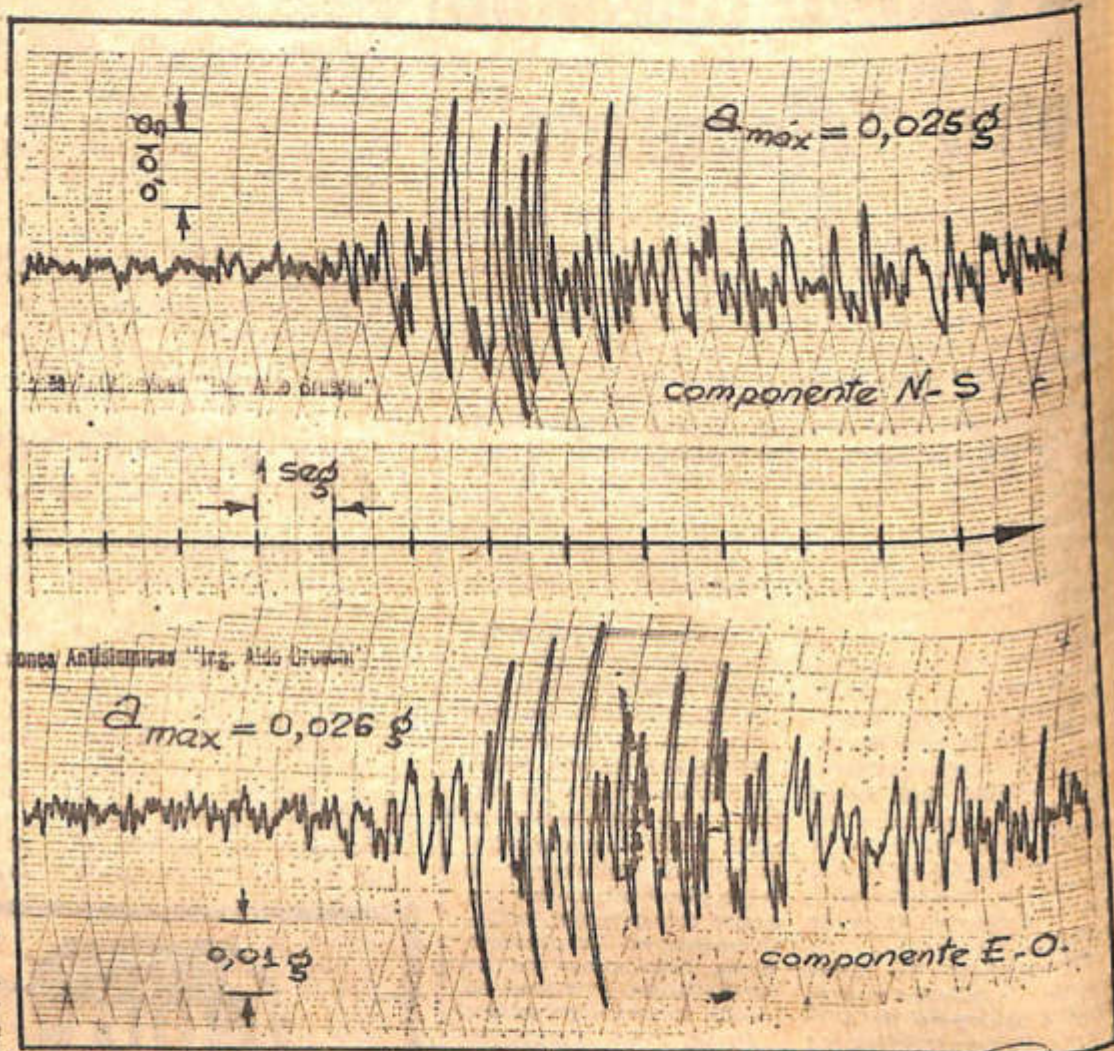
Este es el registro del movimiento sísmico producido ayer en las primeras horas de la tarde, logrado con un sismógrafo de fabricación sanjuanina e instalado en el Instituto de Investigaciones Antisísmicas "Ing. Bruschi", de la UNSJ.
